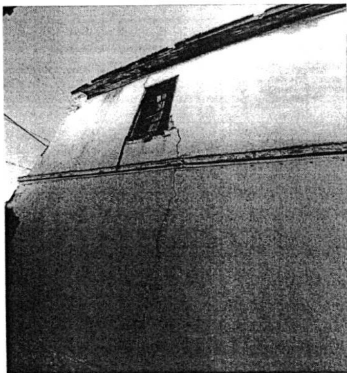
Φωτ 3 κατακόρυφη διαμπερής ρωγμή στην πλάγια όψη
